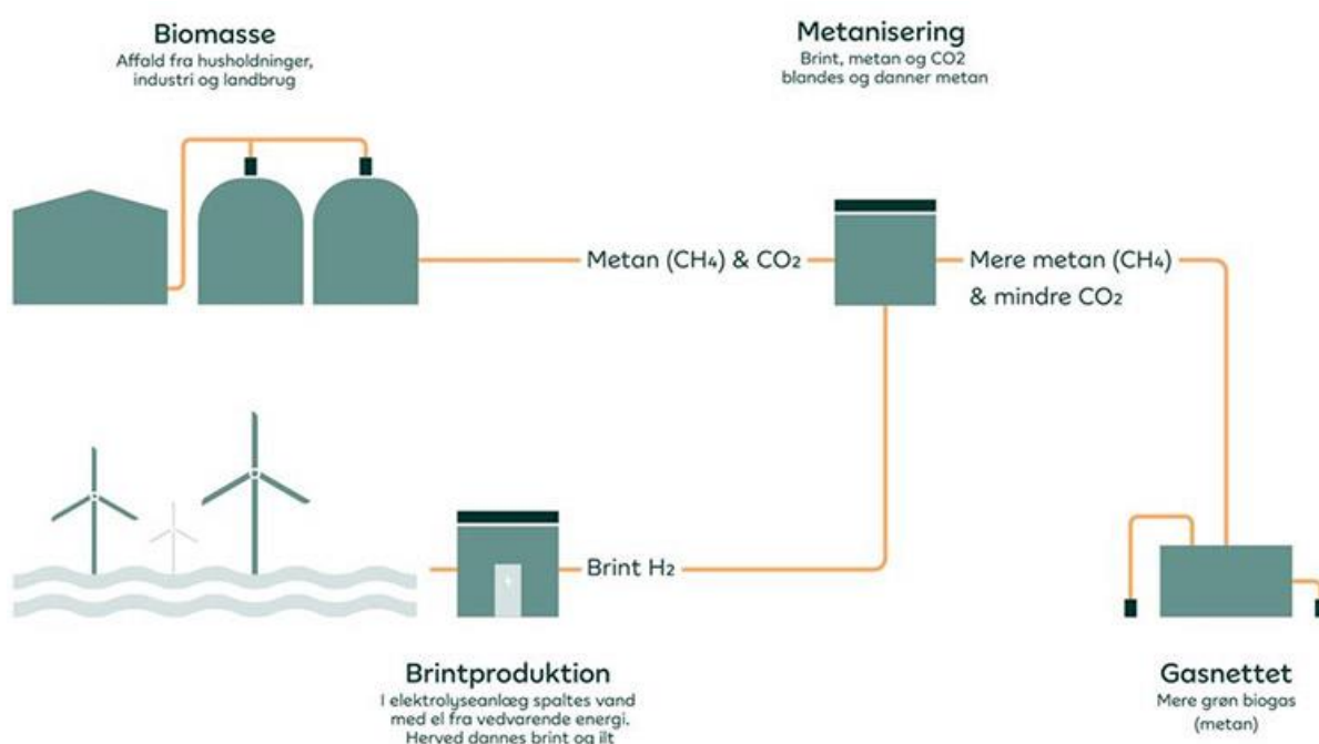
Figur 14: Princippet i metanisering. Fra Nature Energy
